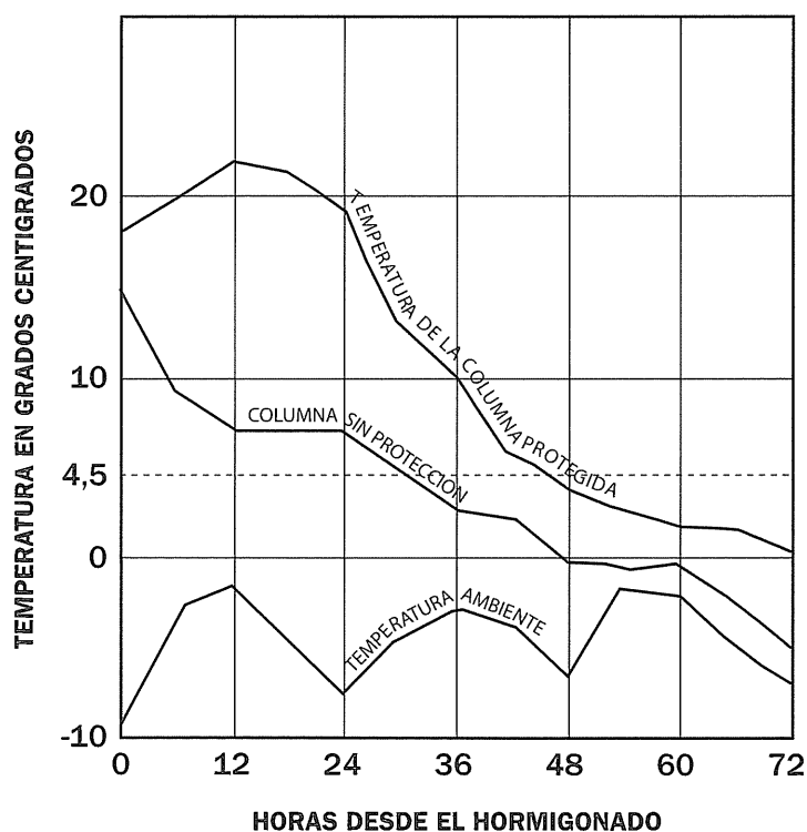
Pérdida de temperatura del hormigón por la acción del frío, columnas protegidas y sin protección
