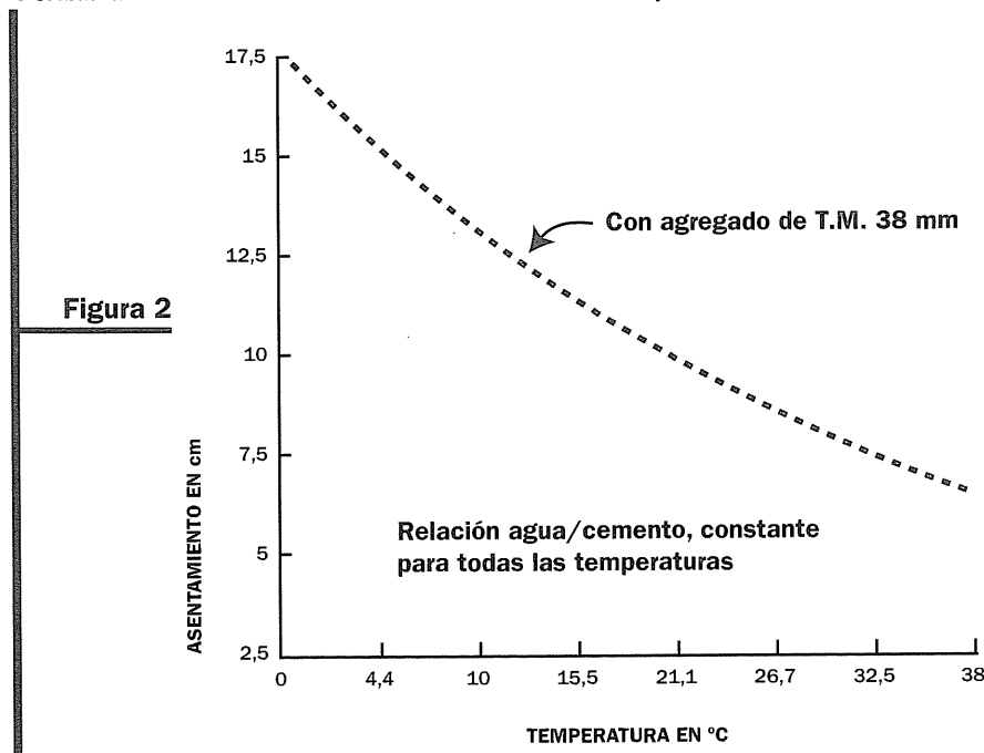
Pérdida de asentamiento debido a la elevación de la temperatura de mezclado
