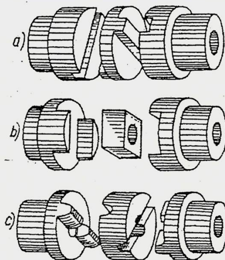
Fig. 12: Acoplamiento Oldham
