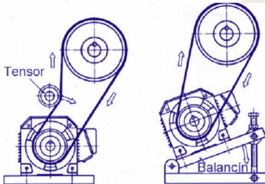
PLACA OSCILANTE
