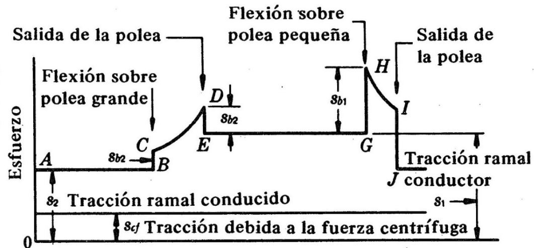
Fig. 17.2 Variación del esfuerzo sobre la correa. Modelo simplificado. (Se- gún W. S. Worley [17.3] )
