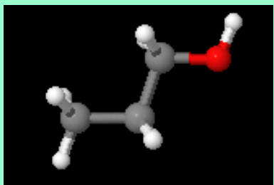
1-propanol
