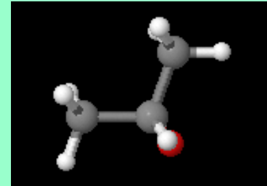
2-propanol
