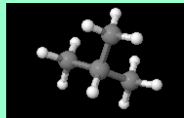
Metilpropano
