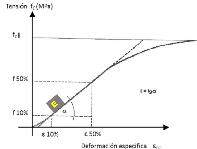
Diagrama de Tensión-Deformación Específica para la determinación de la resistencia a compresión paralela a las fibras.
