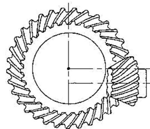
DENTADO HIPOIDAL
