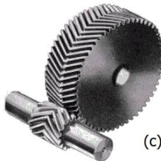
Figura 8 Engranaie Chevron
