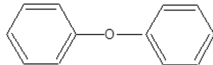
Difeniléther
