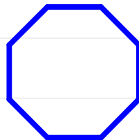
Ciclooctano
