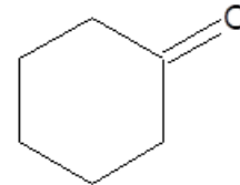
CICLOHEXANONA
