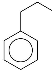
(n)-propilbenceno
