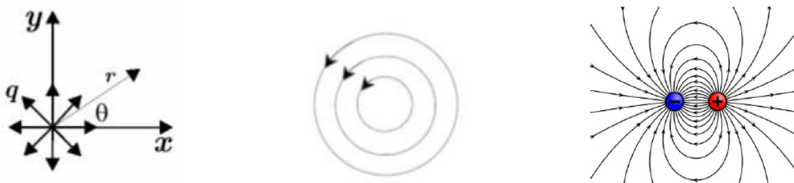
Figura 1. Fuente, vórtice y dipolo (superposición de fuente y sumidero separados una distancia dada).
