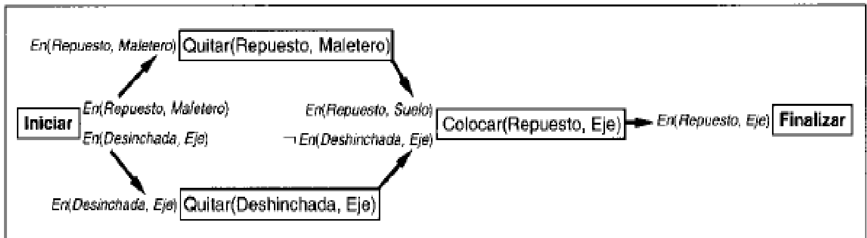
Figura 11.10 La solución final al problema de la rueda de repuesto. Notemos que Quitar(Repuesto, Maletero) y Quitar(Deshinchada, Eje) , puede ser hecho en cualquier orden si son completados antes con la acción Colocar(Repuesto, Eje) .
