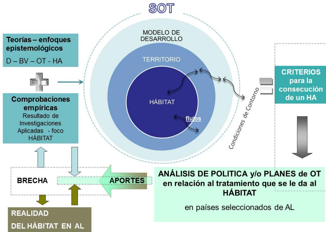
Gráfico Nº 1: esquema metodológico
