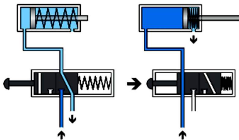
Cilindros de simple efecto
