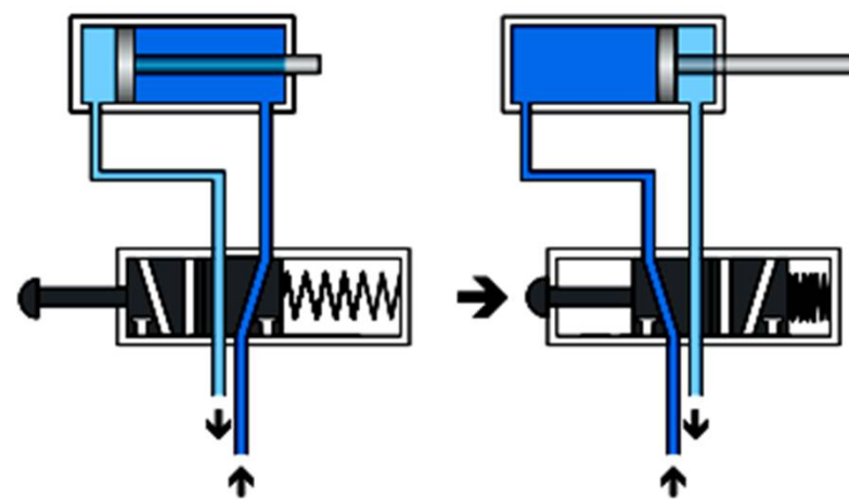
Cilindros de doble efecto
