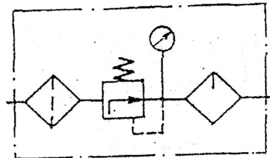
Filtro - Regulador - Lubricador
