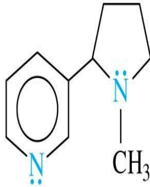
nicotina en el tabaco
