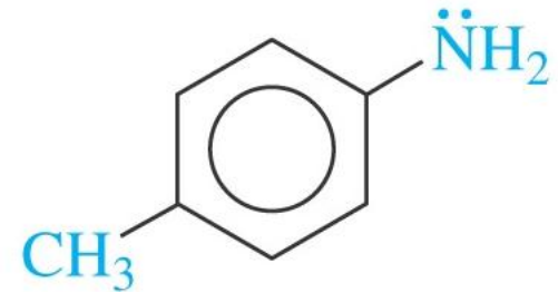
4-metilanilina o p-toluidina
