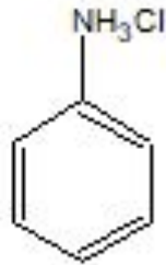
Cloruro de anilinio (Clorhidrato de anilina)
