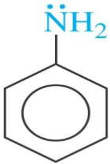
Anilina o Benzenamina
