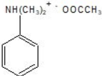
Acetato de N,N-dimetilanilinio
