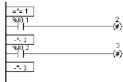
Grafcet Ladder
