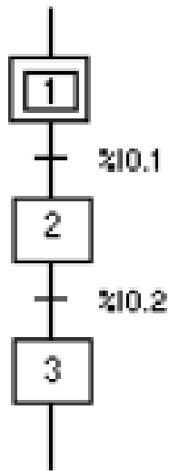
Grafcet gráfico
