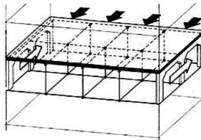
Diafragma rígido
