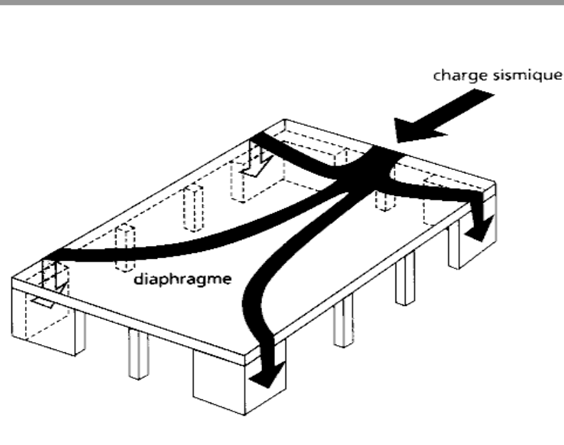
Transmisión de acciones sísmicas por diafragmas
