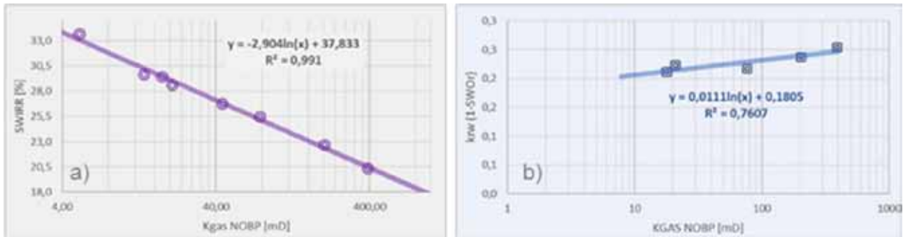
Figura 8. Puntos extremos correlacionados con la permeabilidad. a) Swirr; b) Kwr.
