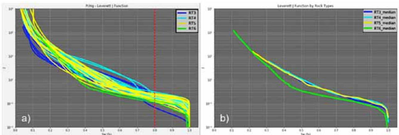
Figura 11. a) Funciones J estimadas de presiones capilares. b) Selección por rocktype.
