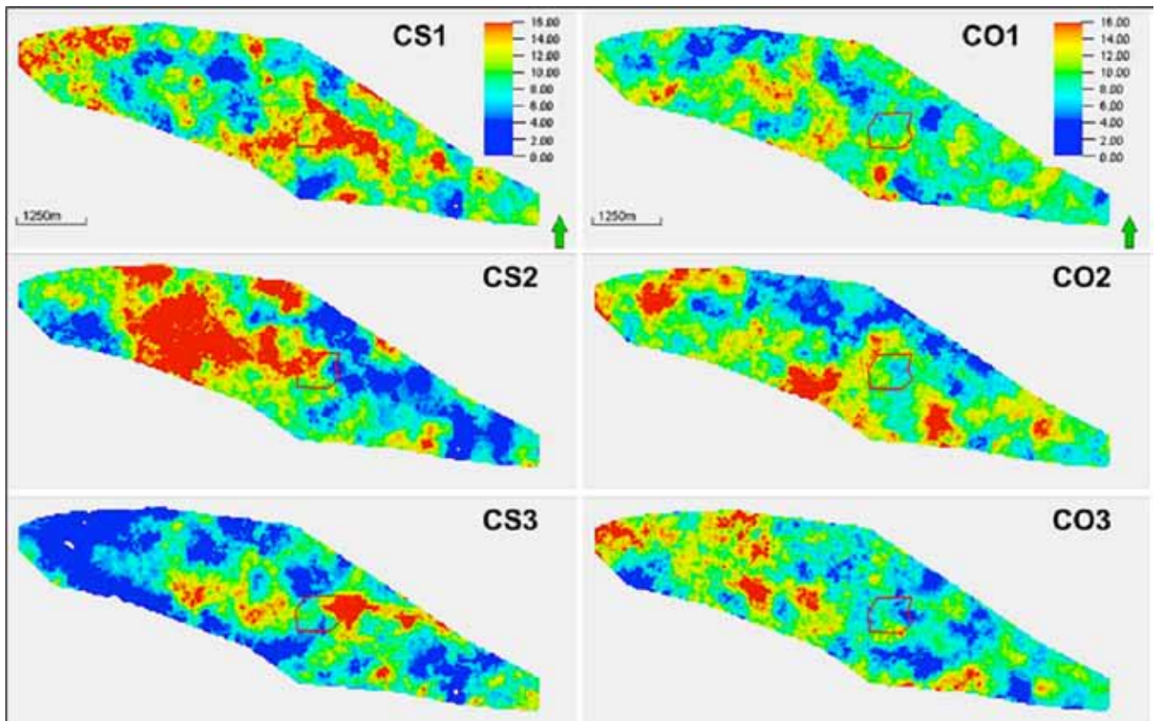
Figura 4. Espesores [m] de facies reservorio (Facies 2, 3, 4 con cutoff de 0,1 mD). A la izquierda CS ciclos CS1, CS2 y CS3 | A la derecha CO ciclos CO1, CO2 y CO3. Polígono rojo corresponde al proyecto Piloto.
