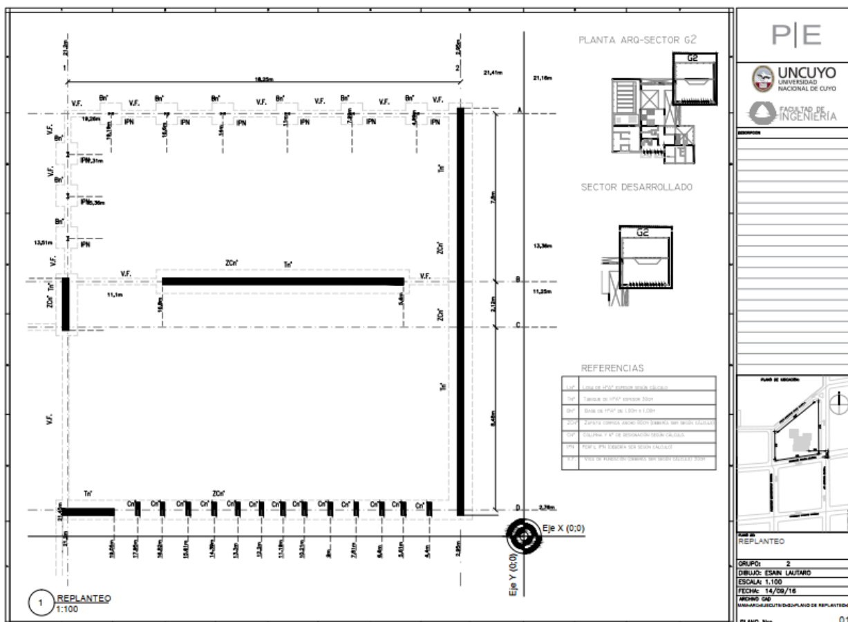
Imagen 2. Plano horizontal desde punto de replanteo por sector.
