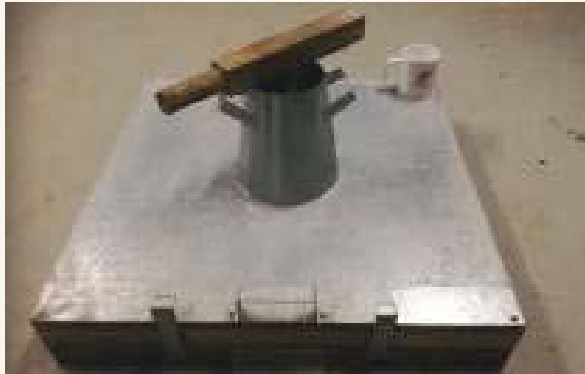
Instrumental para determinar consistencia en Mesa de Graf
