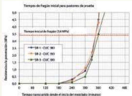
➤ Gráfico de Tiempo inicial de fragüe
