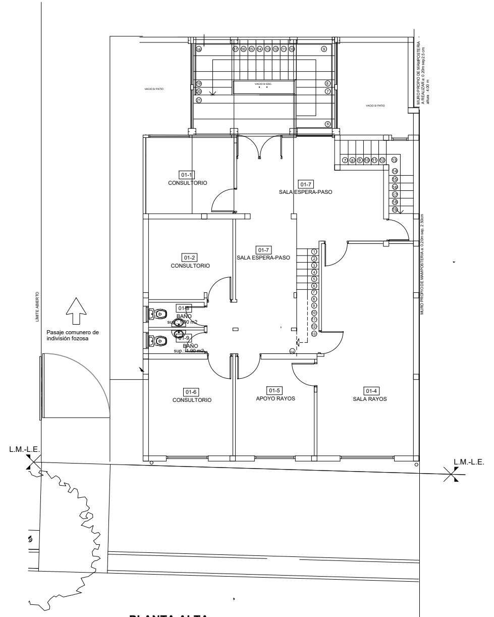
PLANTA ALTA
