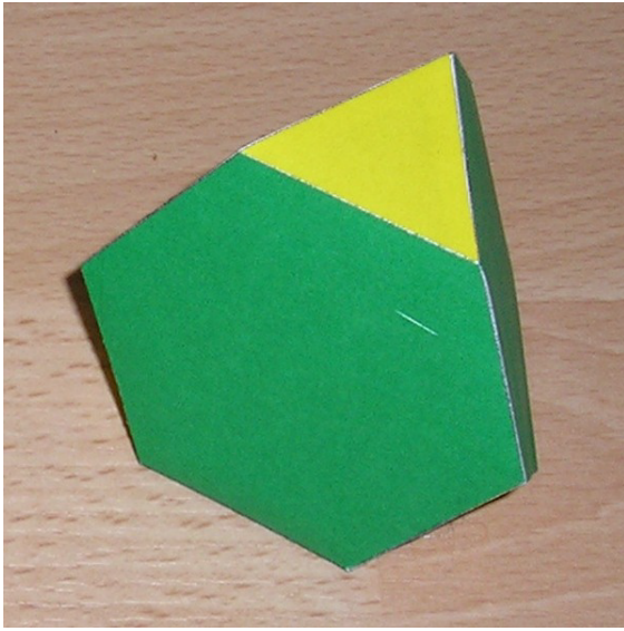
TETRAEDRO TRUNCADO
