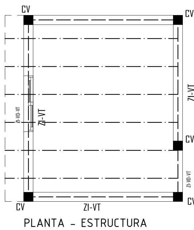
PLANTA - ESTRUCTURA
