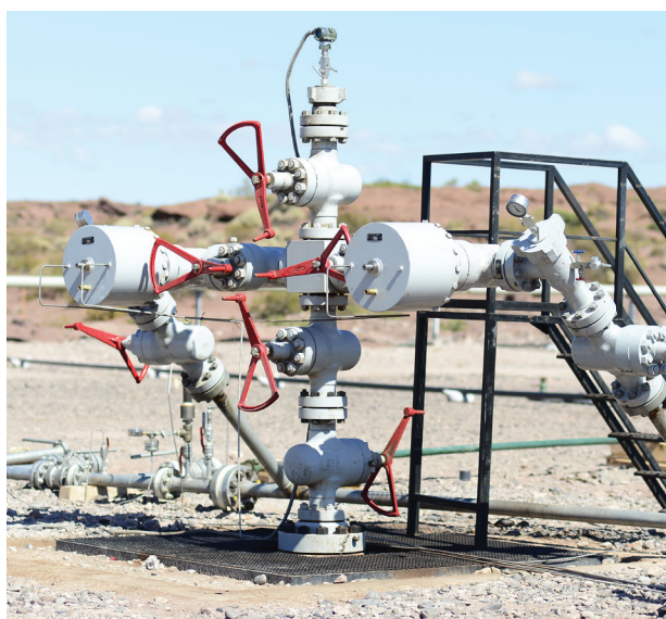
Parte de un "árbol de navidad". Se aprecian las válvulas para controlar el pozo
