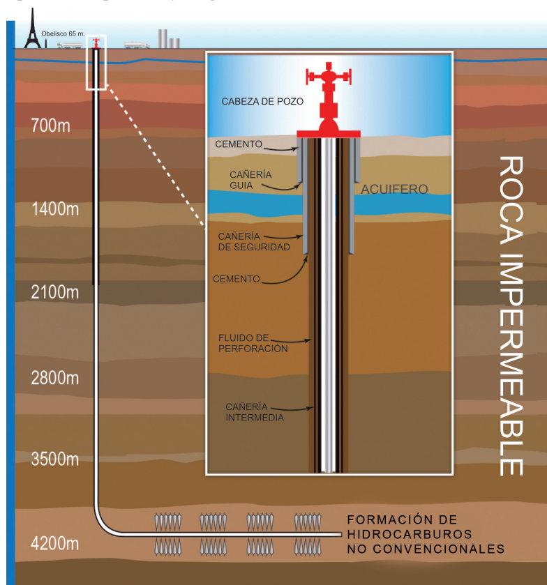
Esquema de un pozo horizontal con detalle del encamisado
