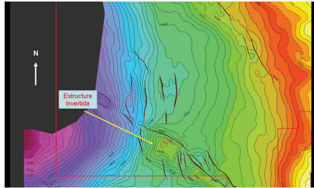
Una imagen generada a partir de trabajos de sísmica
