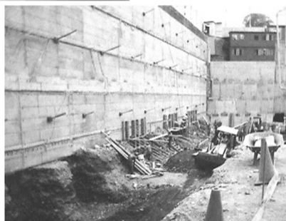
Figura 9.64. Instalación de anclajes para reforzar el talud, unidos mediante vigas de hormigón armado para que trabajen de forma solidaria, Asturias (foto L. González de Vallejo).
