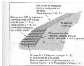
Figura 9.52. Estabilización de un talud mediante escollera.
