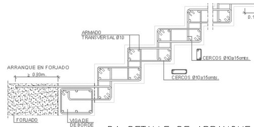
D1 DETALLE DE ARRANQUE
