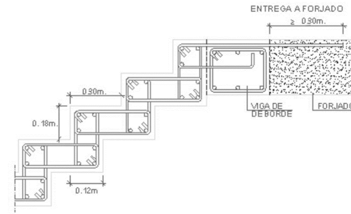
D2 DETALLE DE ENTREGA
