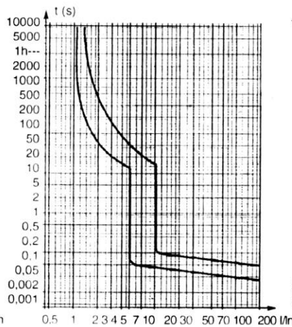
Curva "C"
