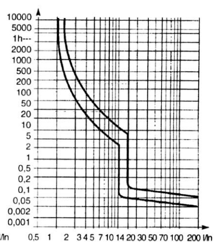
Curva "D"
