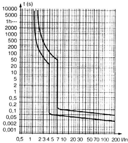
Curva "B"
