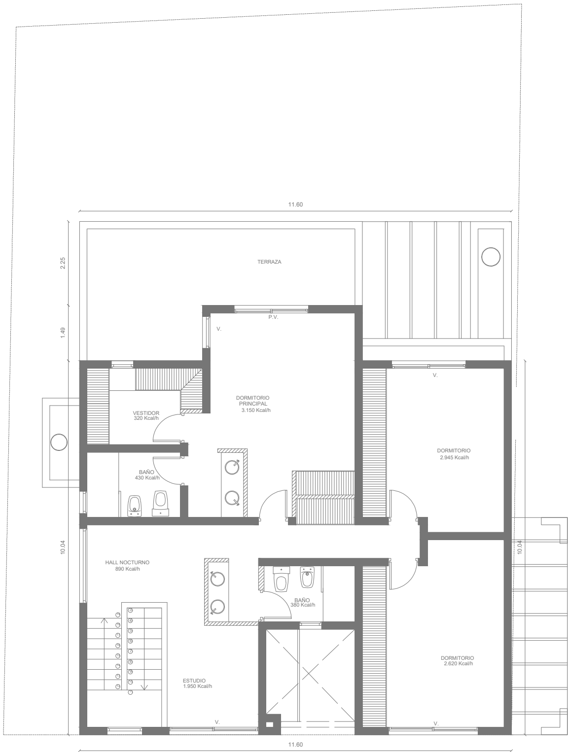
PLANTA ALTA E: 1:100
