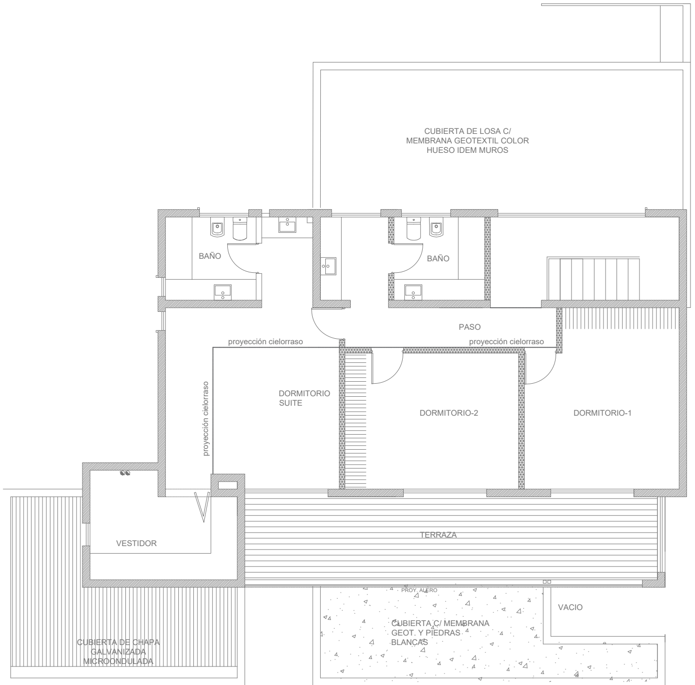
Planta alta E: 1:100
