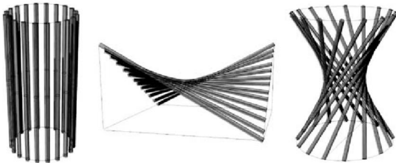
Superficies regladas: cilindro, paraboloid hiperbólico, hiperboloide.
