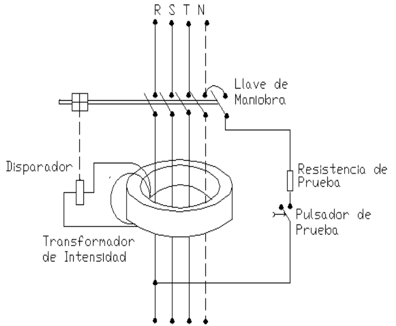
Interruptor Diferencial
