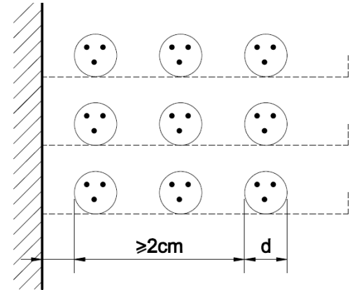
b) Disposición sobre bandeja perforada
