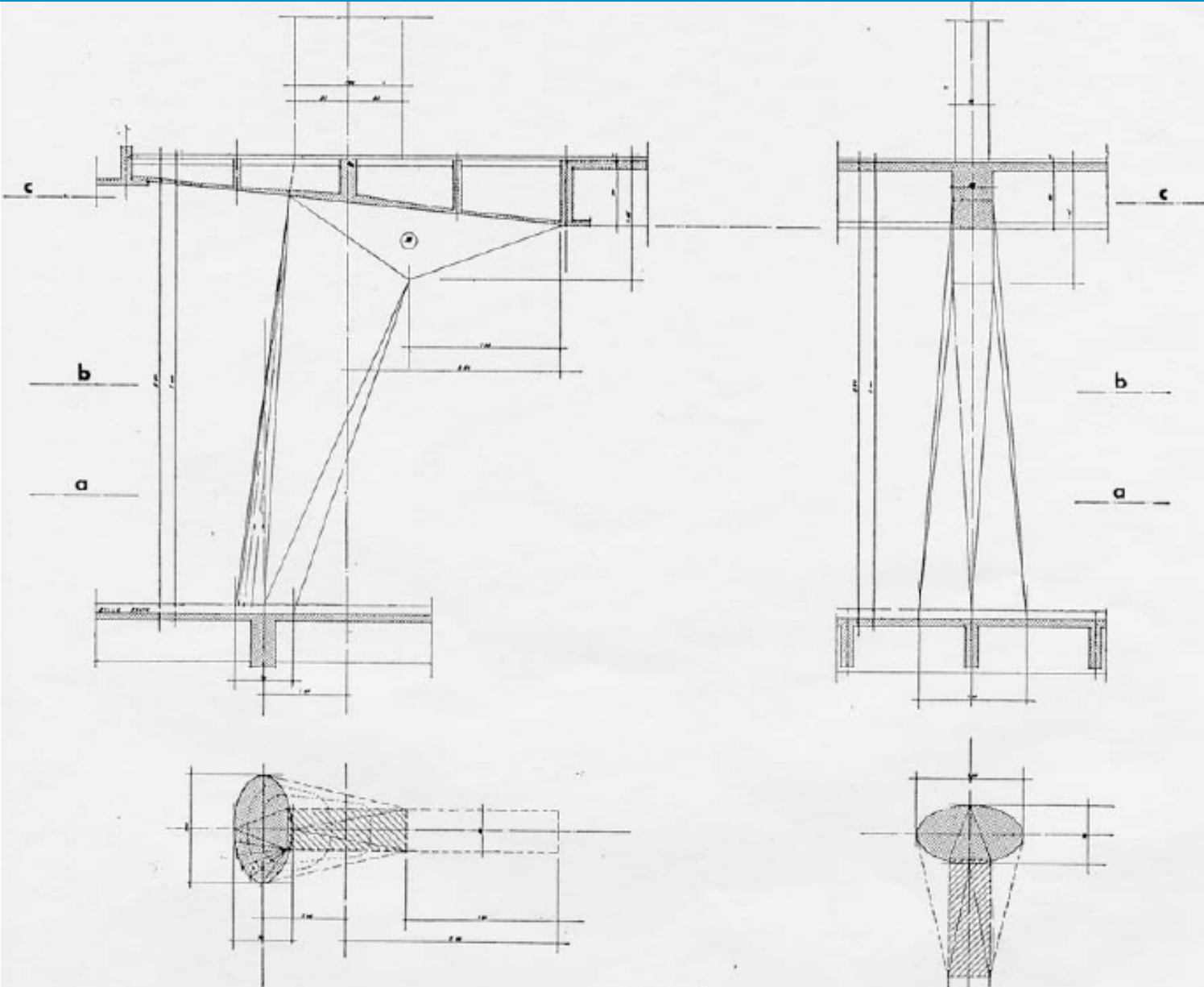
Base de sección elíptica cuyo eje mayor se dispone paralelo al edificio
