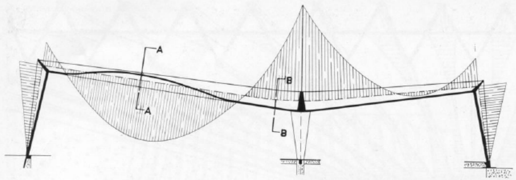
DIAGRAMA DE MOMENTOS
