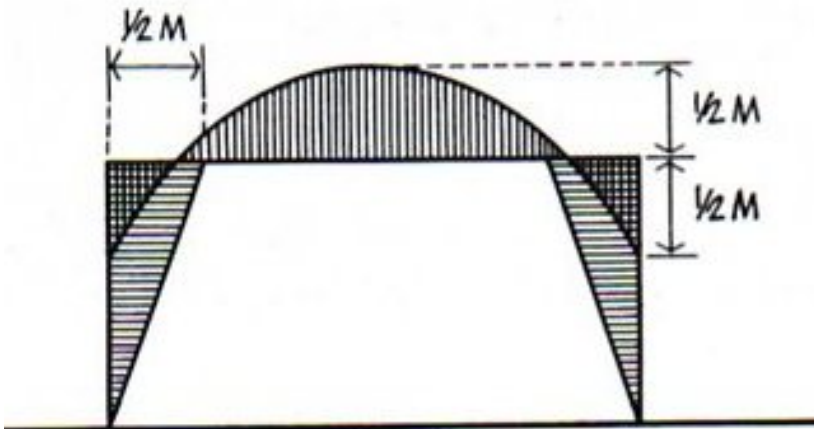
TENSIONES DE FLEXION
