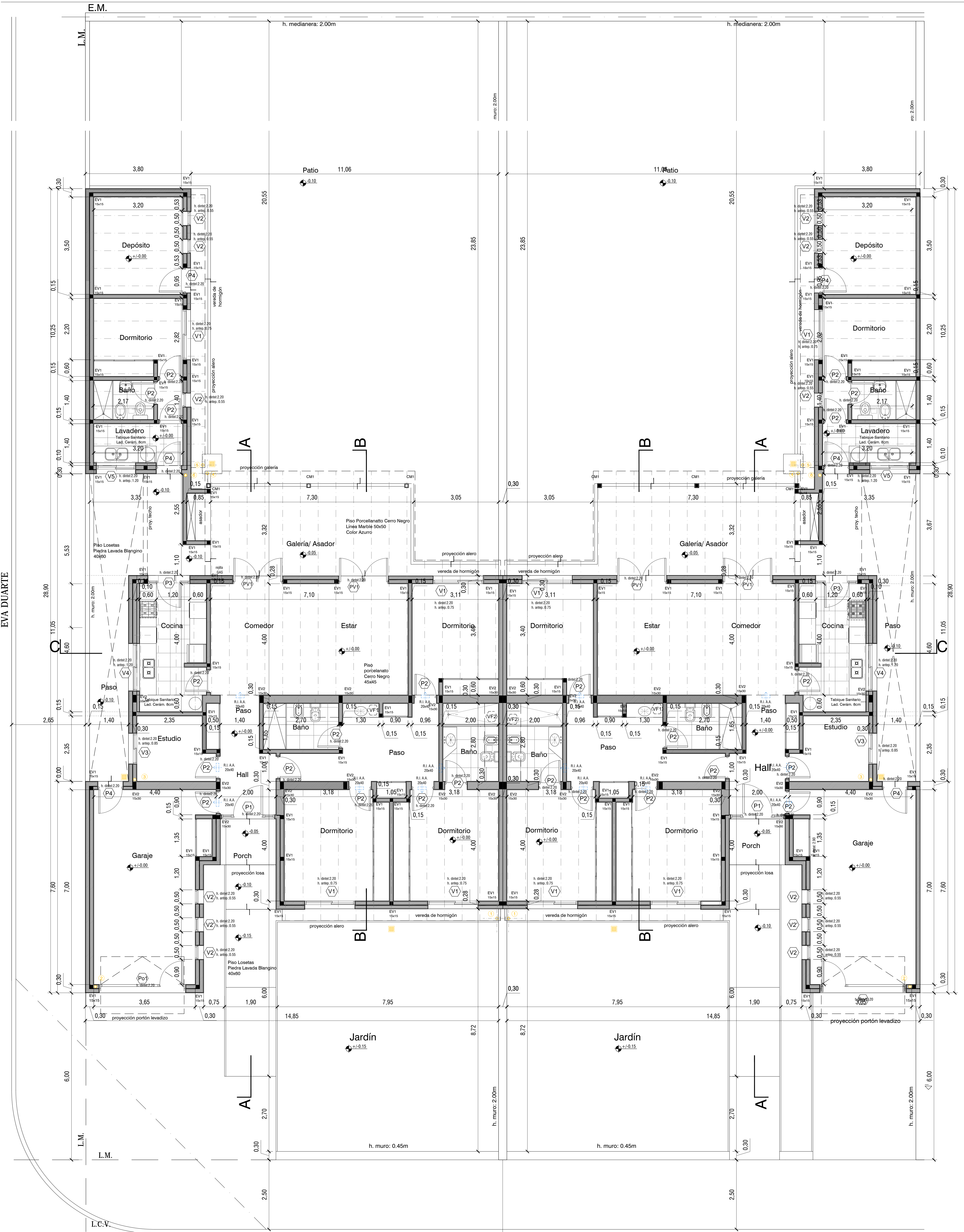
PLANTA GENERAL
