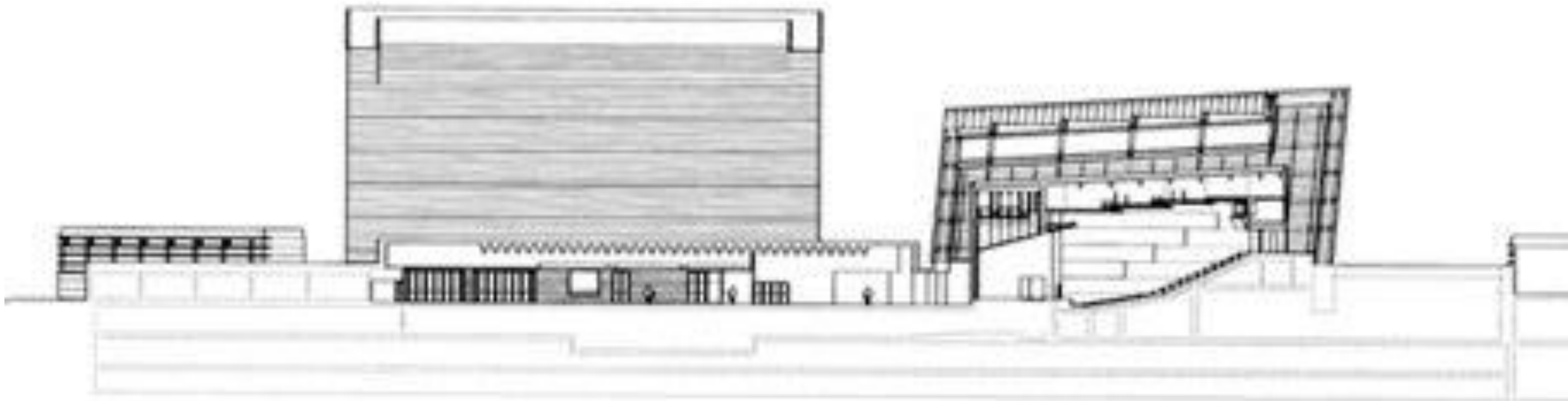
VISTA- CORTE AUDITORIO Y SALA CAMARA (la planta Auditorio y los cortes y vistas están en la misma escala)
