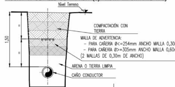
FIGURA 1: DETALLE DE TAPADA (S/ NOTA IMPORTANTE N°3)
