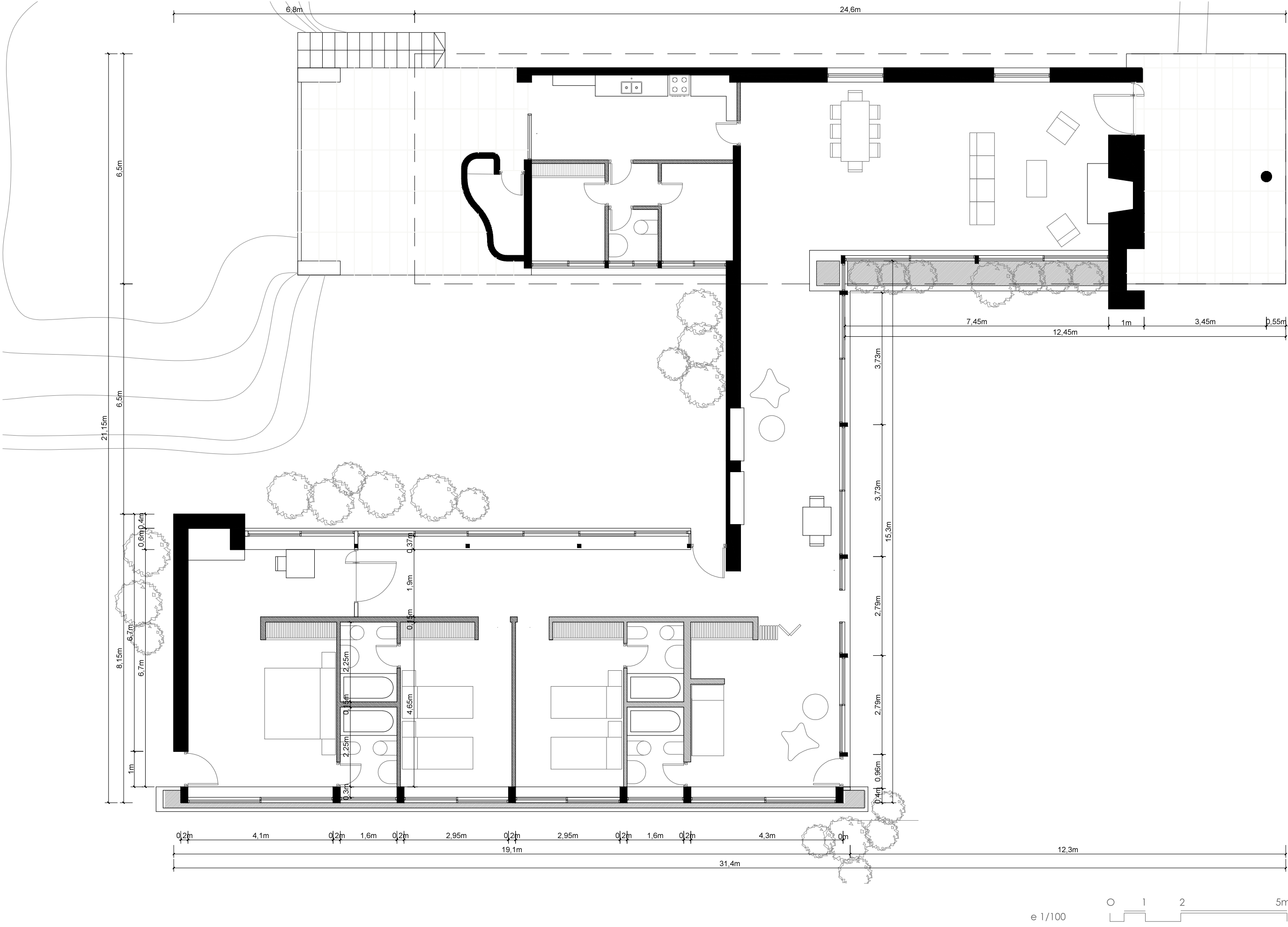
PLANTA
