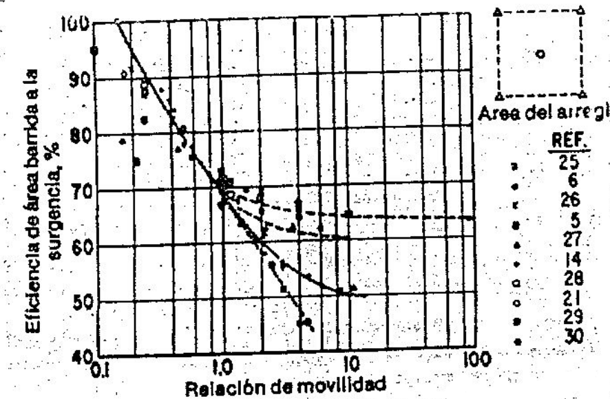
Fig.7: Eficiencia de barrido para un arreglo desarrollado (tomado de Craig 4 )
