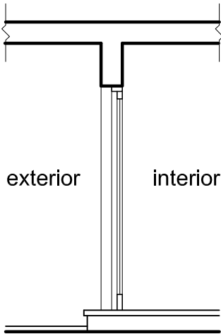
PUERTA-VENTANA CORREDIZA
