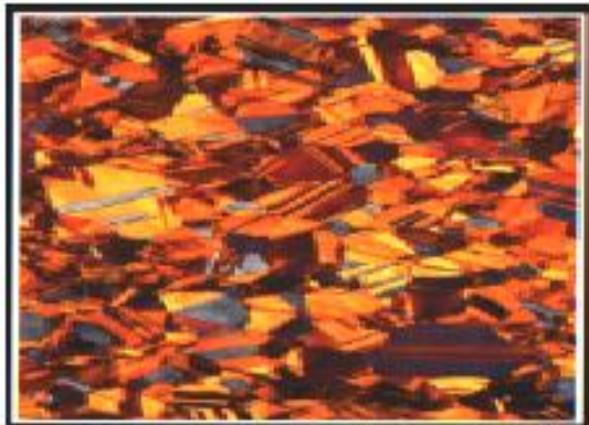
Micrografia óptica de un latón policristalino. 100X.
