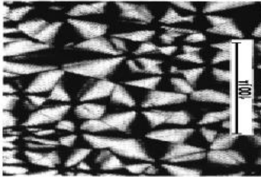
Micrografia óptica de transmisión de un polietileno de estructura esferulítica. 525X.
