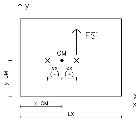
a. Fuerza sísmica Y con e+
