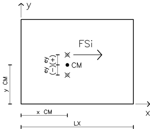
a. Fuerza sísmica X con e+
