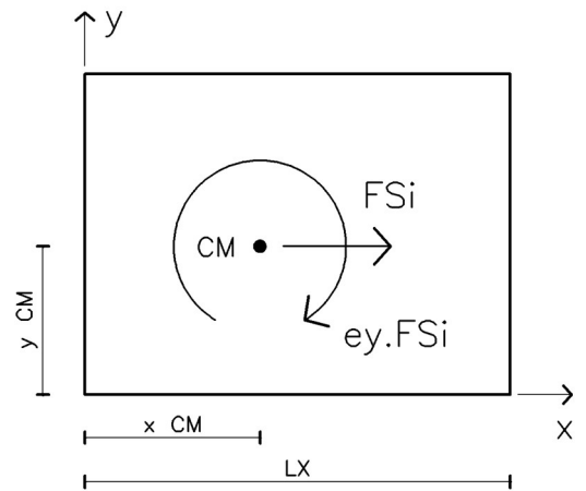
b. Cargas para aplicar en el modelo
