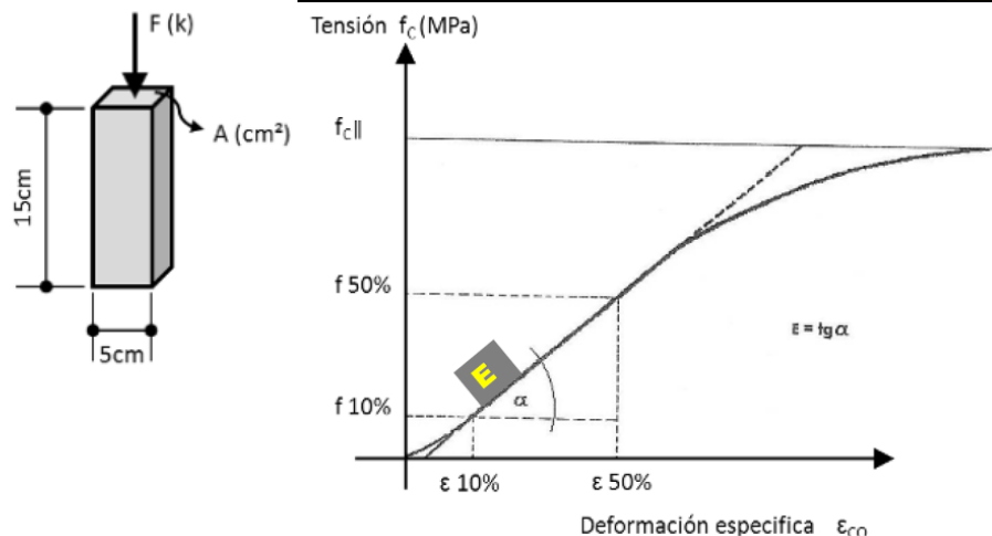
Diagrama de Tensión-Deformación Específica para la determinación de la resistencia a compresión paralela a las fibras.
