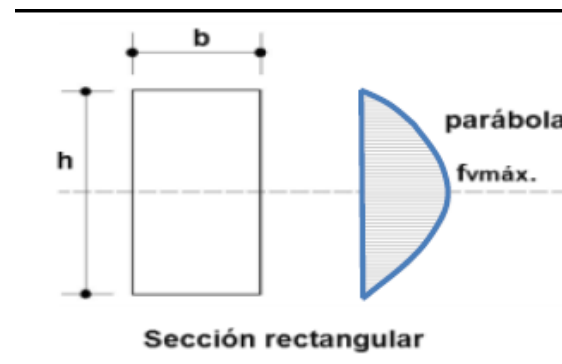
Esfuerzo cortante
