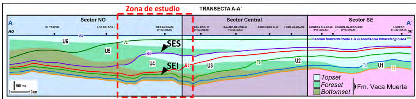
Figura 2. Zona de estudio sobre la transecta A-A' mostrando la sectorización geográfica, las unidades sísmicas y la distribución de los segmentos ( bottomset/foreset/topset ) de clinoformas (modificado de Marchal et al. 2016a). Ubicación de la Sección Enriquecida Inferior (SEI) y de la Sección Enriquecida Superior (SES).
