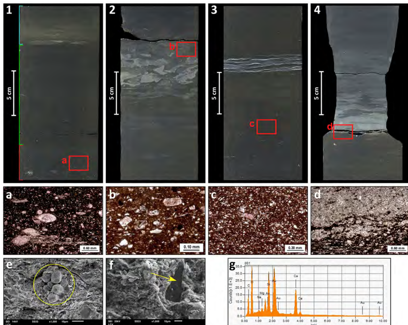
Figura 12. Sección Enriquecida Superior. 1-4 fotos de corona: 1) fangolita fosilífera (llave roja), fangolita algo calcárea (llave verde) y toba piritizada (llave azul); 2 y 4) capas piroclásticas alteradas a calcita o arcilla, parcialmente disturbadas por bioturbación; en algunos casos sólo quedan cristales tamaño arena fina de plagioclasas “flotando” en las fangolitas (foto b, flecha); 3) aspecto masivo de la fangolita. Nótese la abundancia de partículas silicoclásticas tamaño limo (puntos blancos, foto c); a-d) microfotografías de cortes delgados con nicóles paralelos (ubicación de los mismos en fotos de corona 1-4, recuadros rojos): a) fauna relativamente diversa compuesta por radiolarios, foraminíferos y valvas de pelecípodos; d) reemplazo por calcita como mosaico de cristales “sucios”; e-f) microscopía electrónica: e) porosidad intraparticular en framboides de pirita (círculo); f) aspecto de la matriz calcárea. Clasto de cuarzo (flecha); g) espectro analítico de elementos obtenido a partir de un EDS realizado en la matriz de una fangolita calcárea. Los picos más altos corresponden a oxígeno, silicio y calcio.
