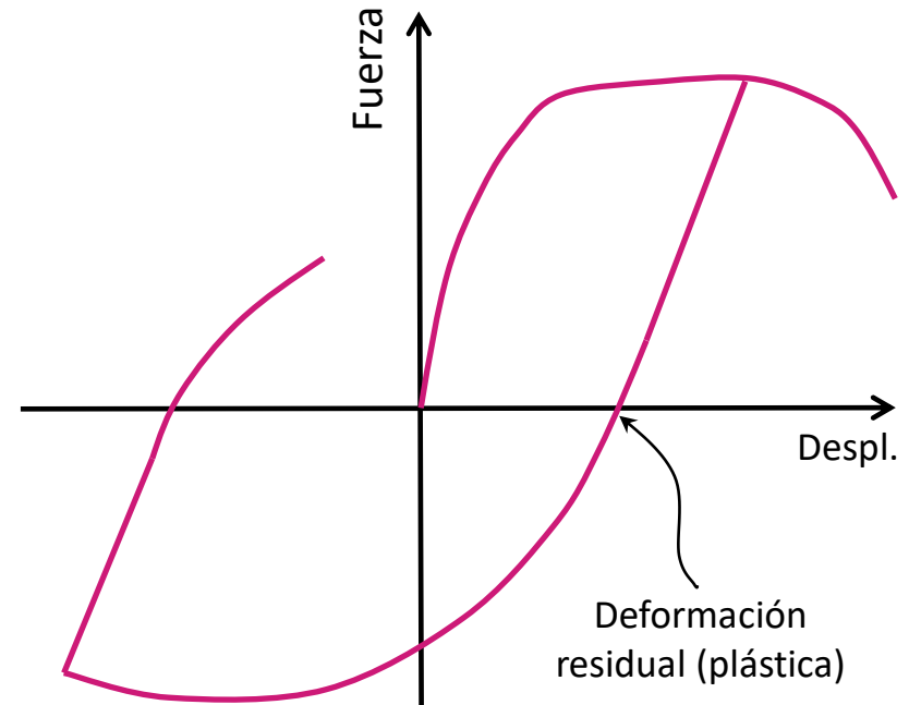
Respuesta no lineal inelástica
